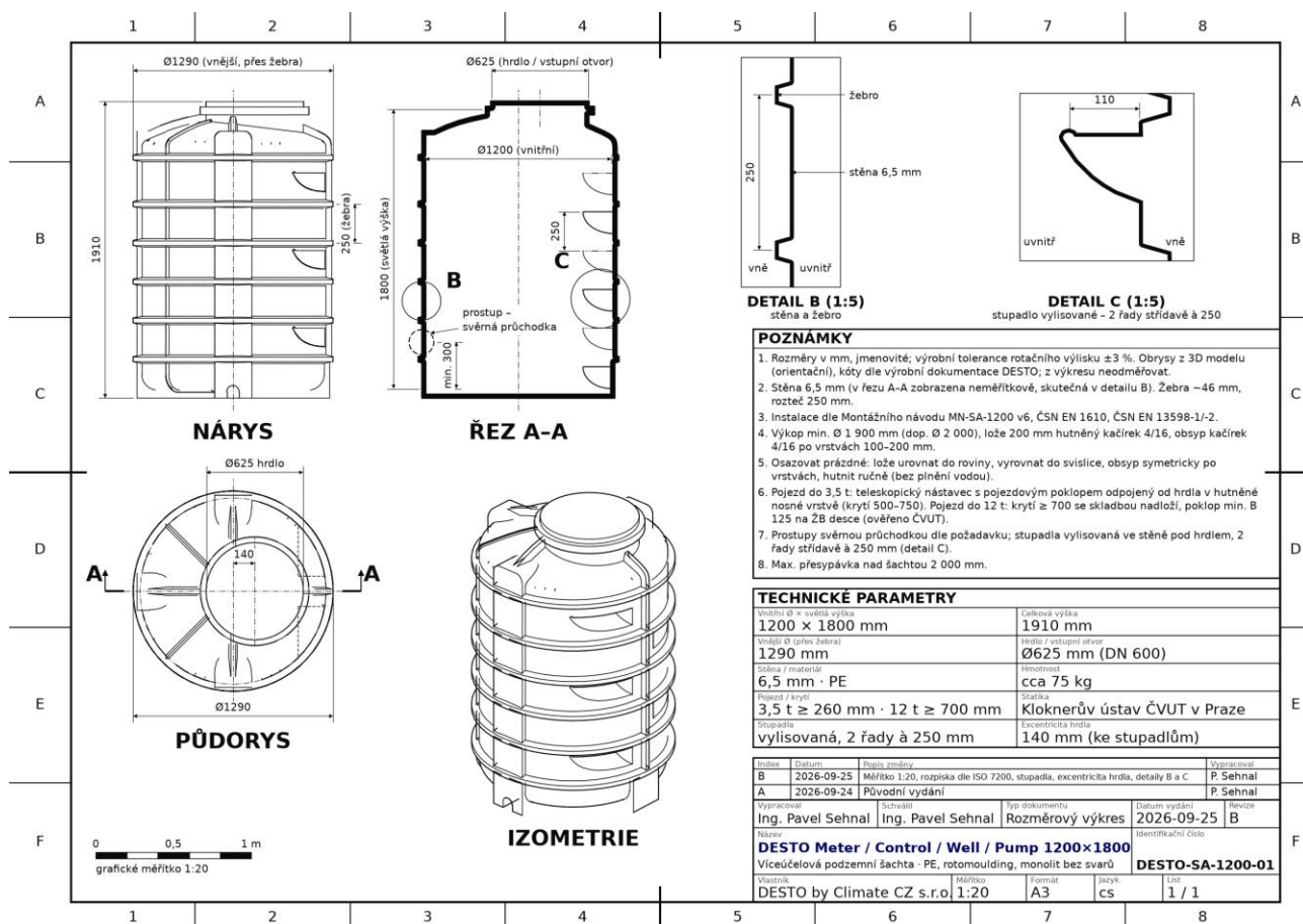
Obr. 1 – Rozměrový výkres DESTO-SA-1200-01 rev. B (1:20; nárys, řez A-A, půdorys, izometrie, detaily stěny a stupadla). Samostatně jako PDF a DXF.
